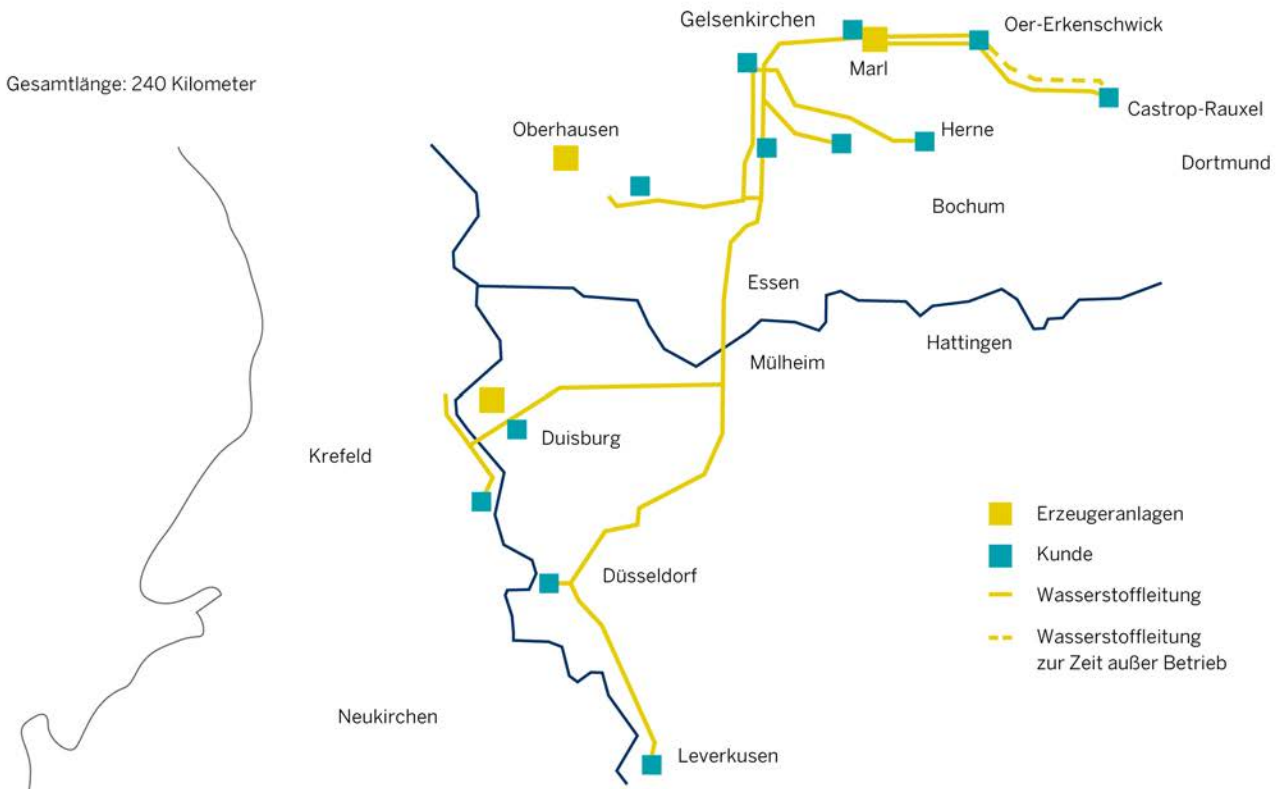
Abbildung 11: Wasserstoffnetz in Nordrhein-Westfalen
